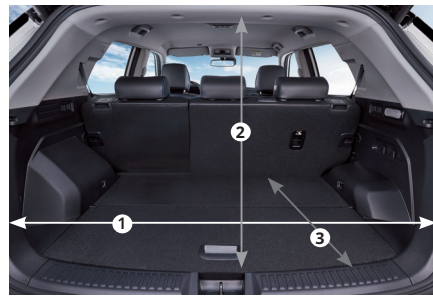
1. Anchura 1.375 mm 2. Altura 935 mm 3. Profundidad 990 mm
